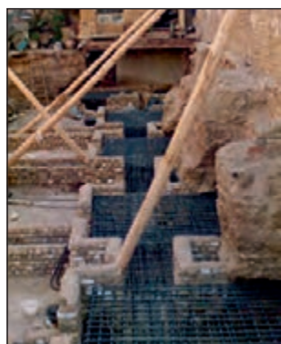
شکل ۹۰-۱ مهاربندی با شمع چوبی
